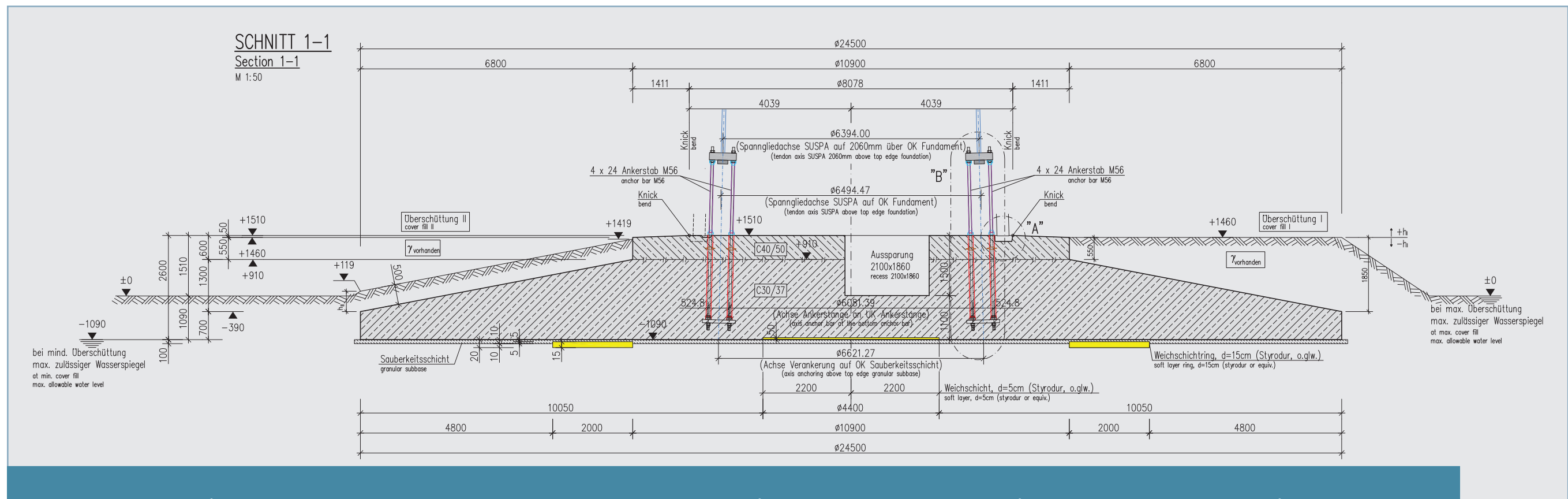
Abb. 1: Schnitt durch das geplante Fundament einer GE 5.3-158 mit 158 m Rotorradius und 229 m Gesamthöhe. Der Durchmesser des Fundamentes beträgt 24,5 m, die Tiefe 2,6 m und das Gewicht rund 1750 Tonnen. Quelle: GE Renewable Energy.
